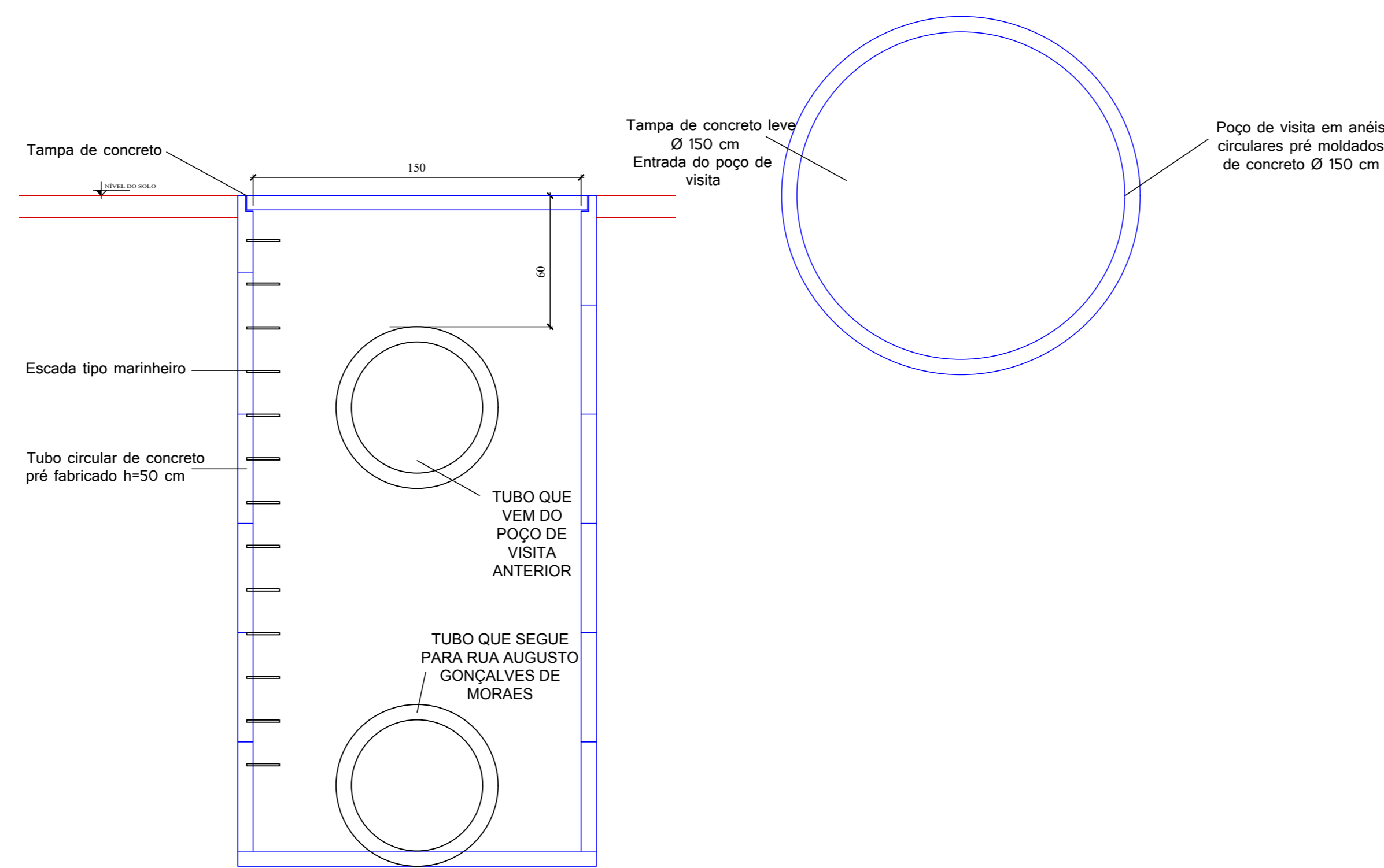
Detalhe poço de visita Esc: 1/20
