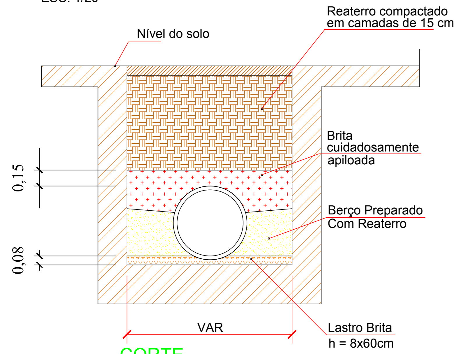
Detalhe assintamento dos tubos de concreto Esc: 1/20
