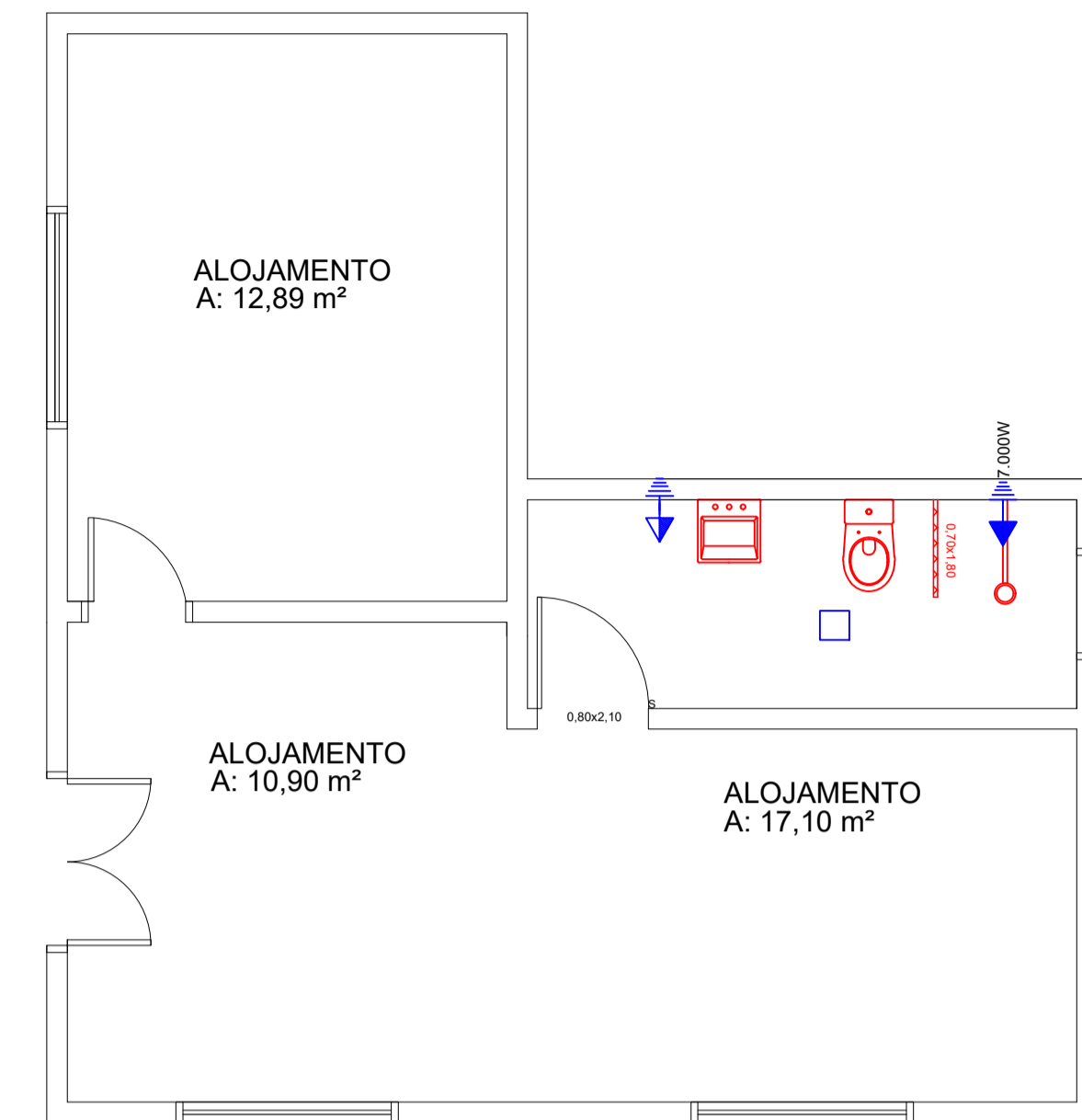
PLANTA BAIXA - PONTOS ELÉTRICOS Escala 1/50
