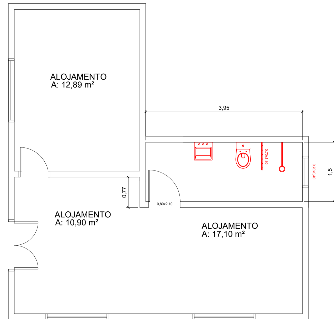
PLANTA BAIXA - TÉRREO ESC.: 1:50
