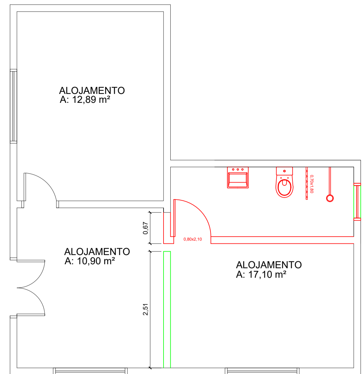
PLANTA BAIXA EXECUTIVA - TÉRREO ESC.: 1:50
