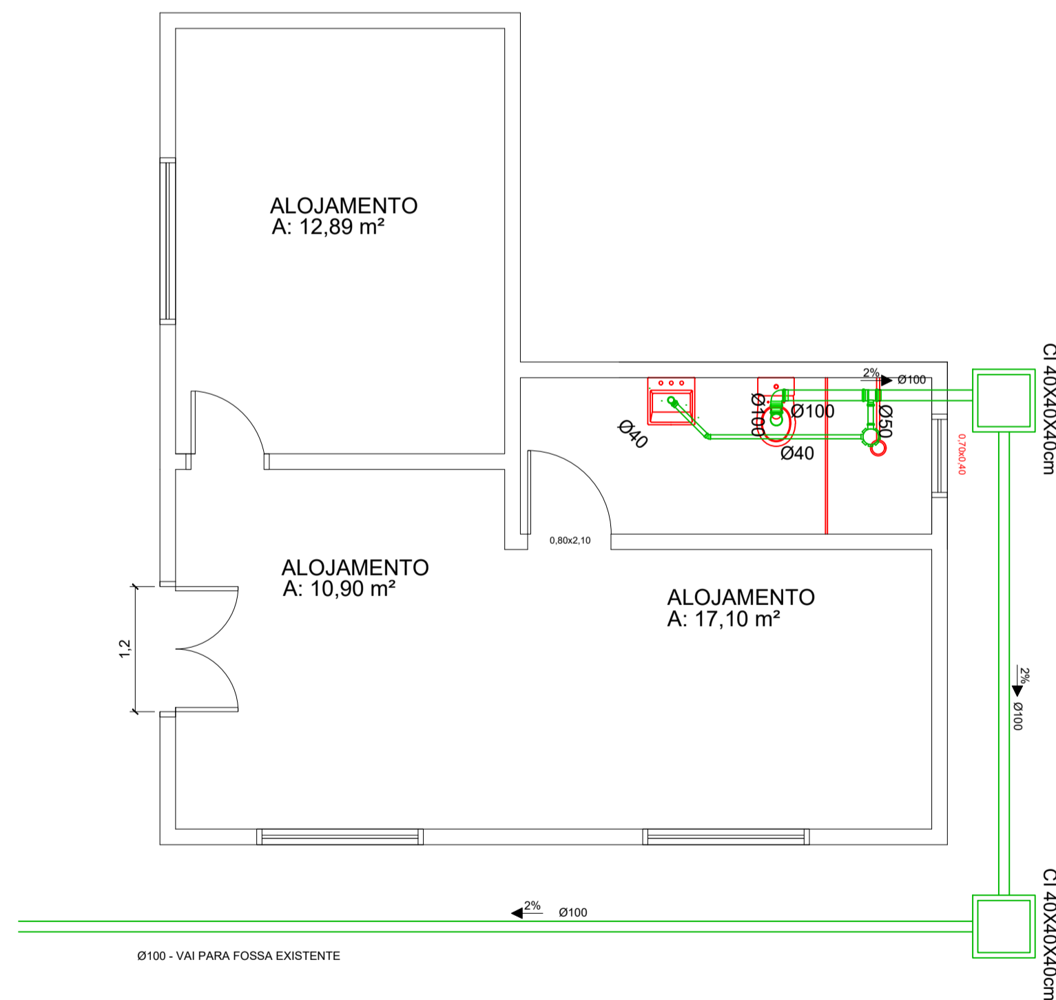
PLANTA BAIXA - SANITÁRIO ESC 1:50
