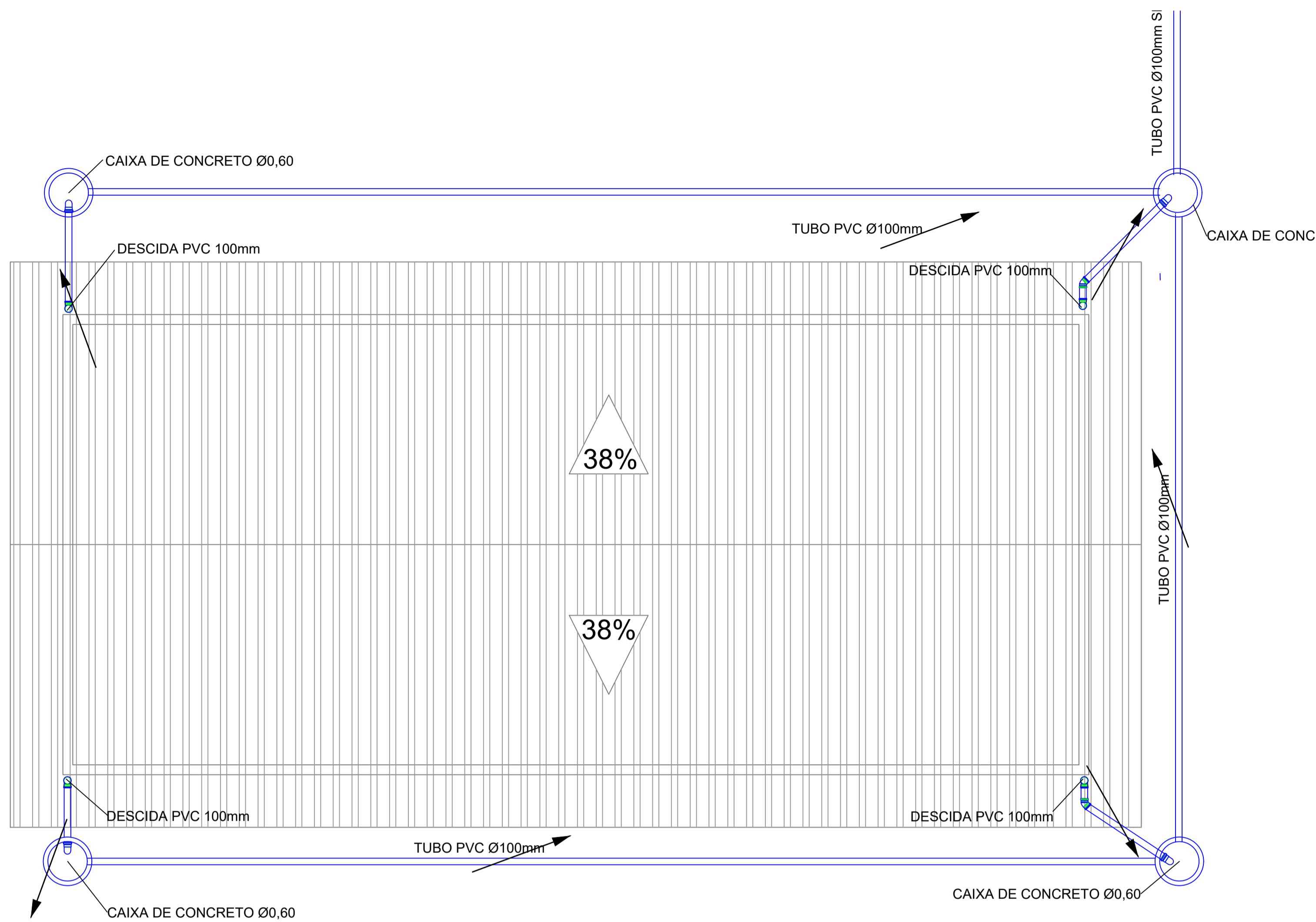
PLANTA ÁGUAS PLUVIAIS ESC 1:50
