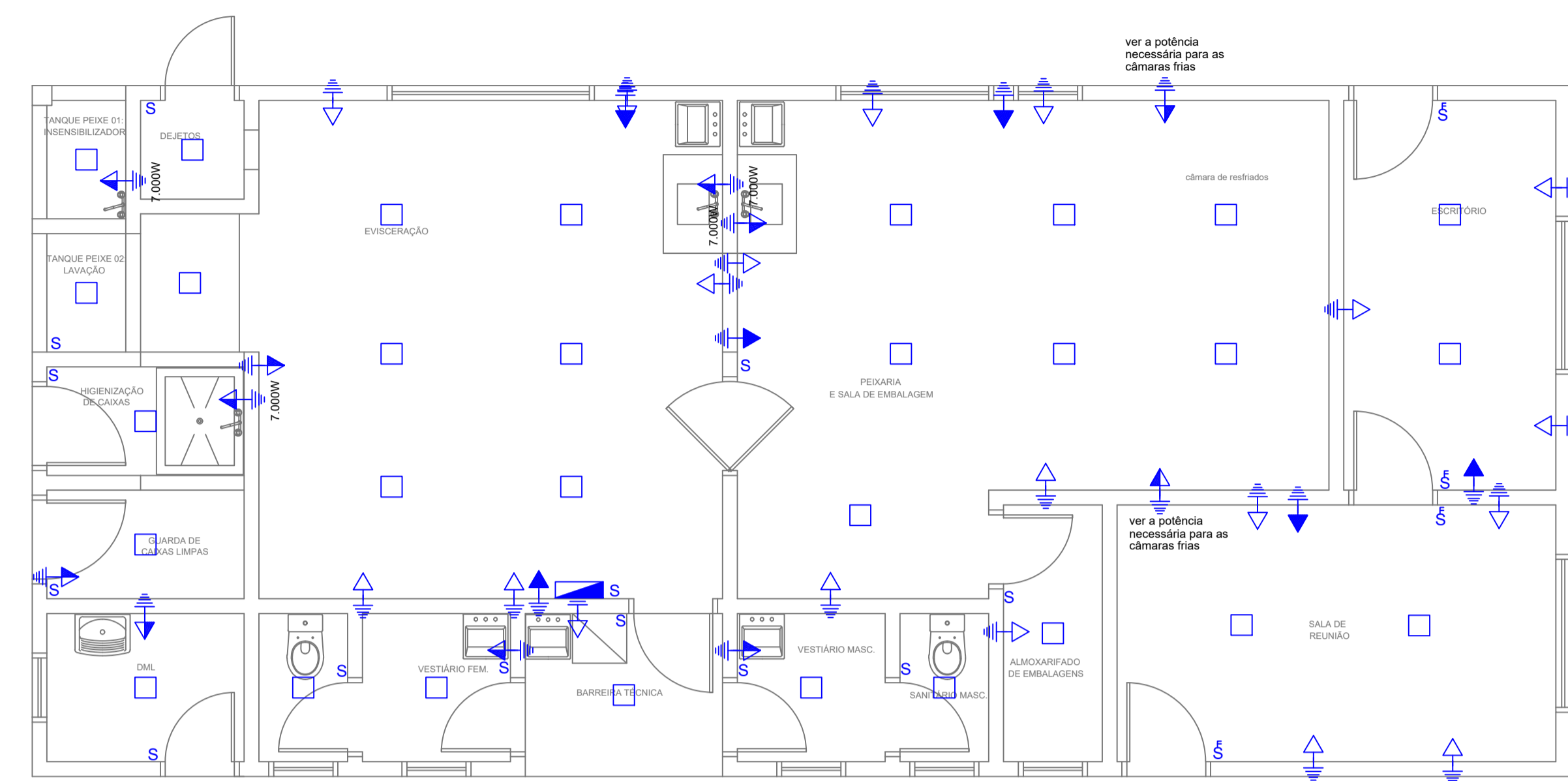
PLANTA BAIXA - PONTOS ELÉTRICOS
