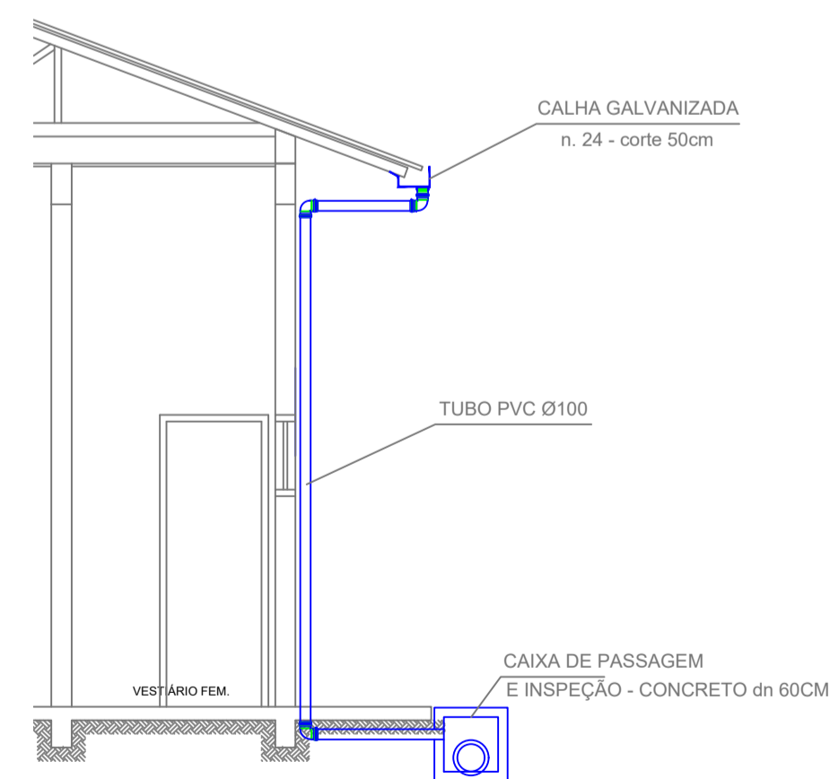
DETALHE DESCIDAS DE ÁGUAS PLUVIAIS ESC 1:50
