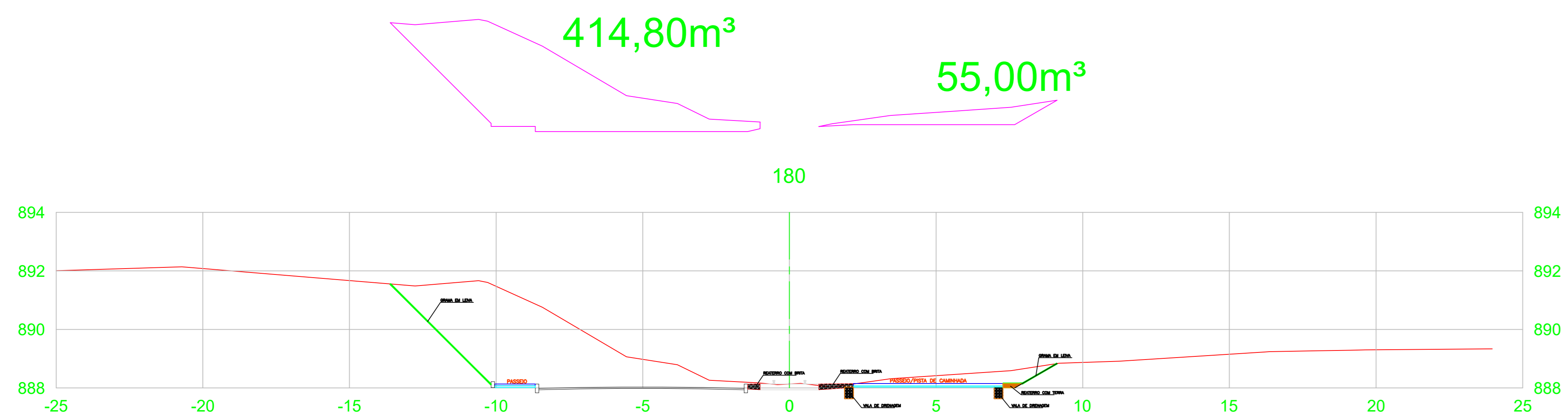
ESTACA 180
