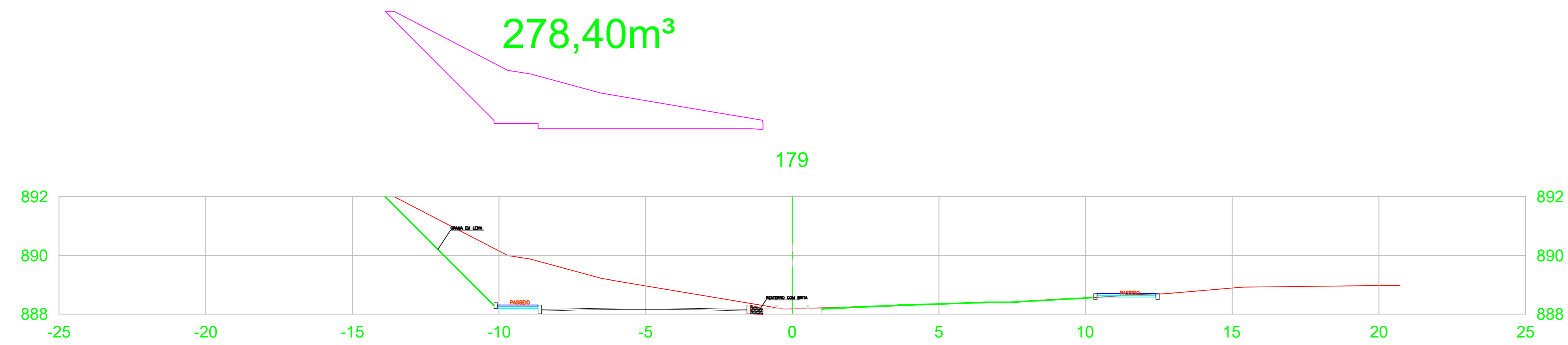
ESTACA 179
