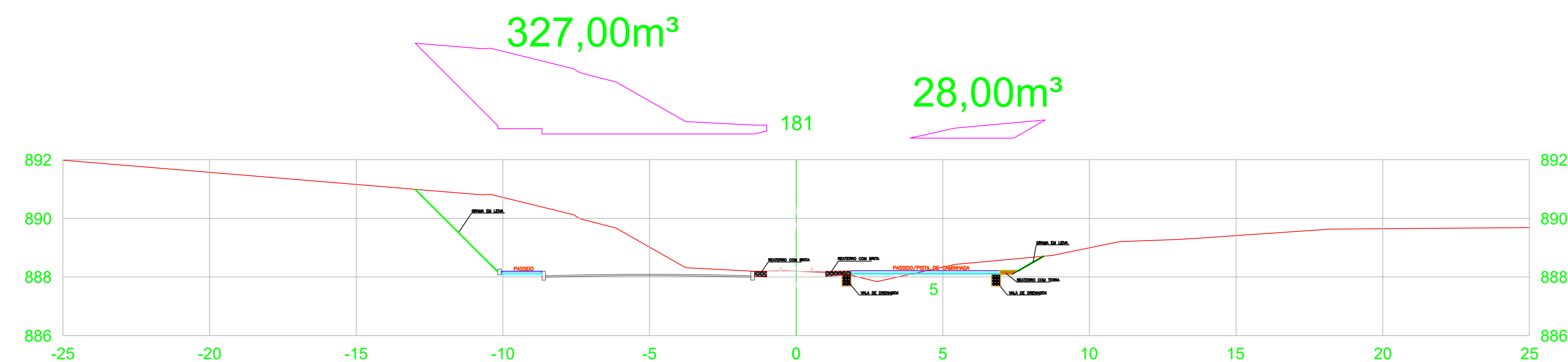
ESTACA 181
