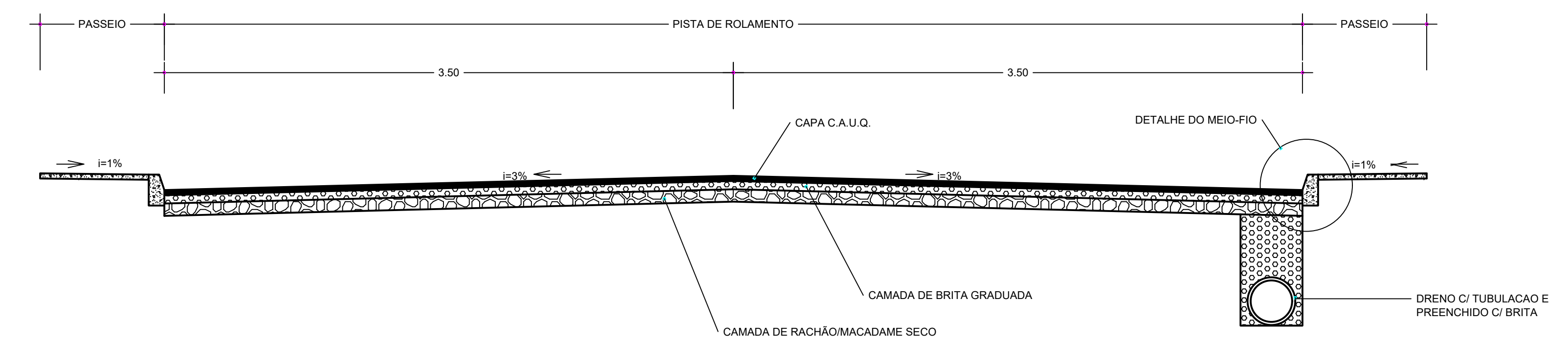
SEÇÃO TRANSVERSAL SEM ESCALA
