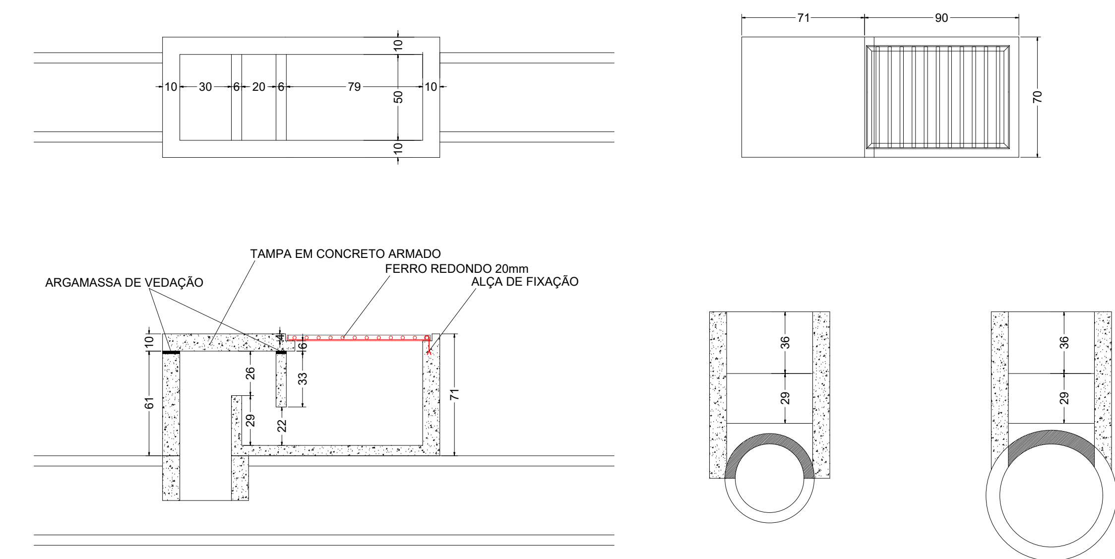
DETALHE DA BOCA DE LOBO ESC. 1/25
