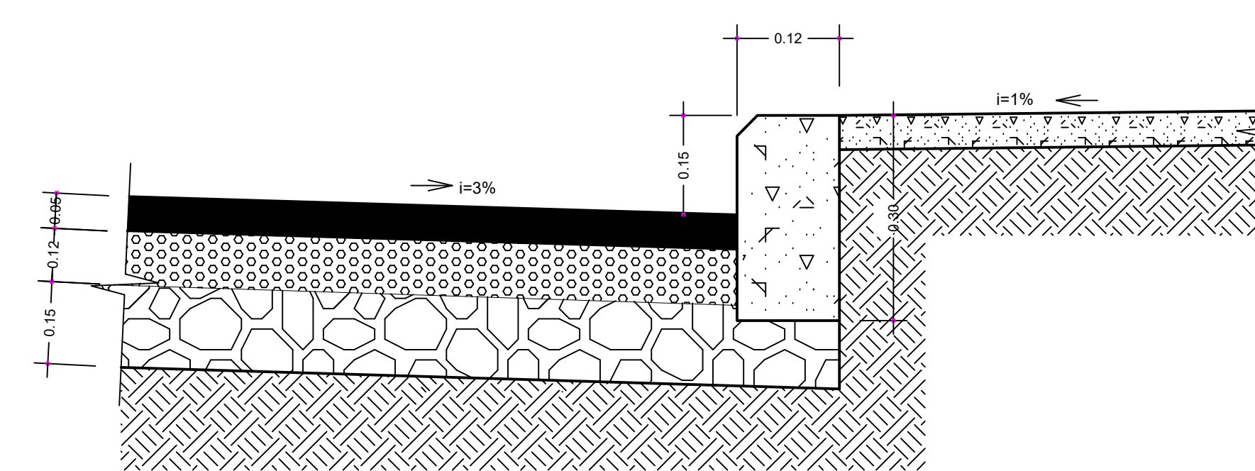
DETALHE DO MEIO-FIO SEM ESCALA
