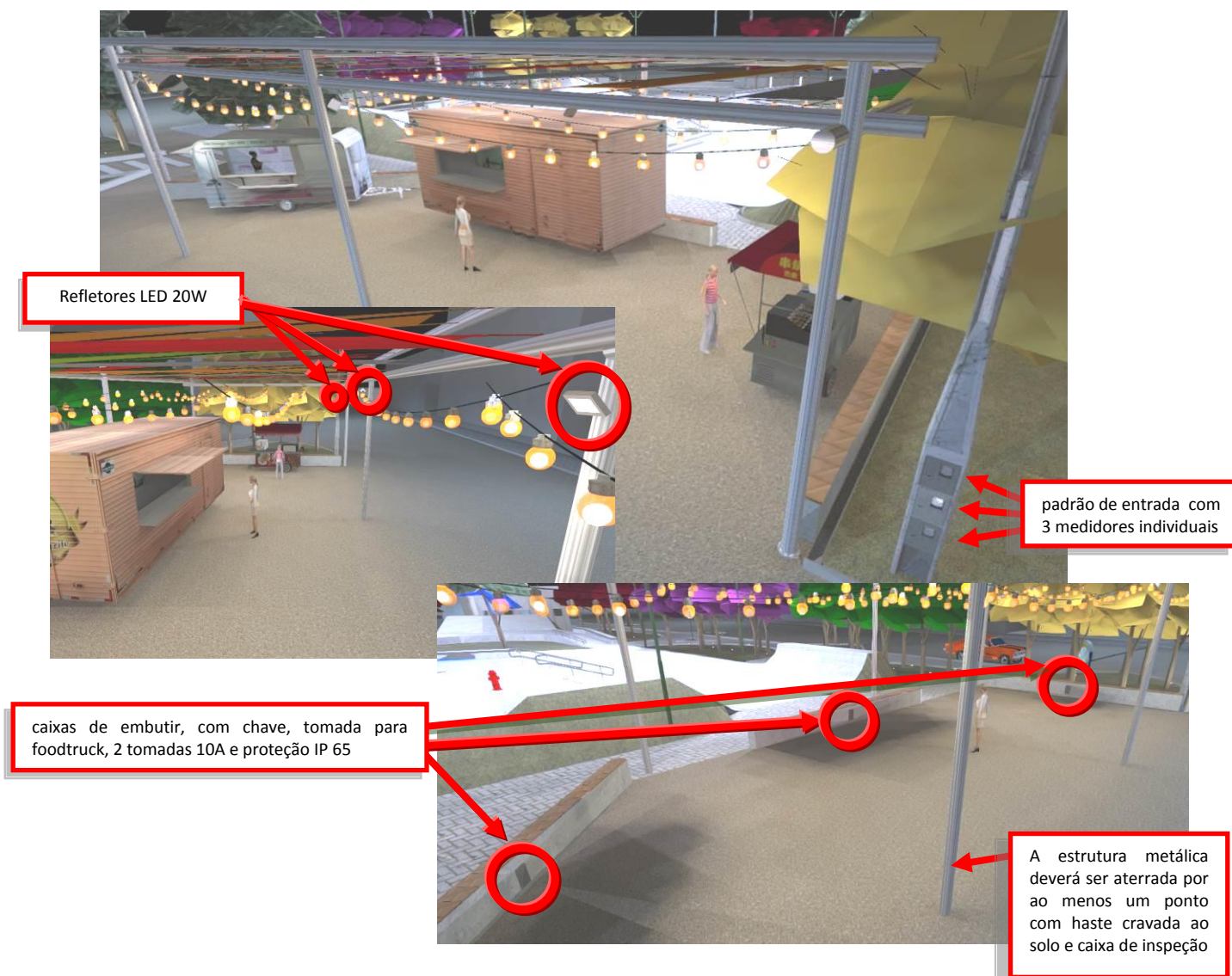
Fig. 11 – Iluminação na área dos foodtrucks
