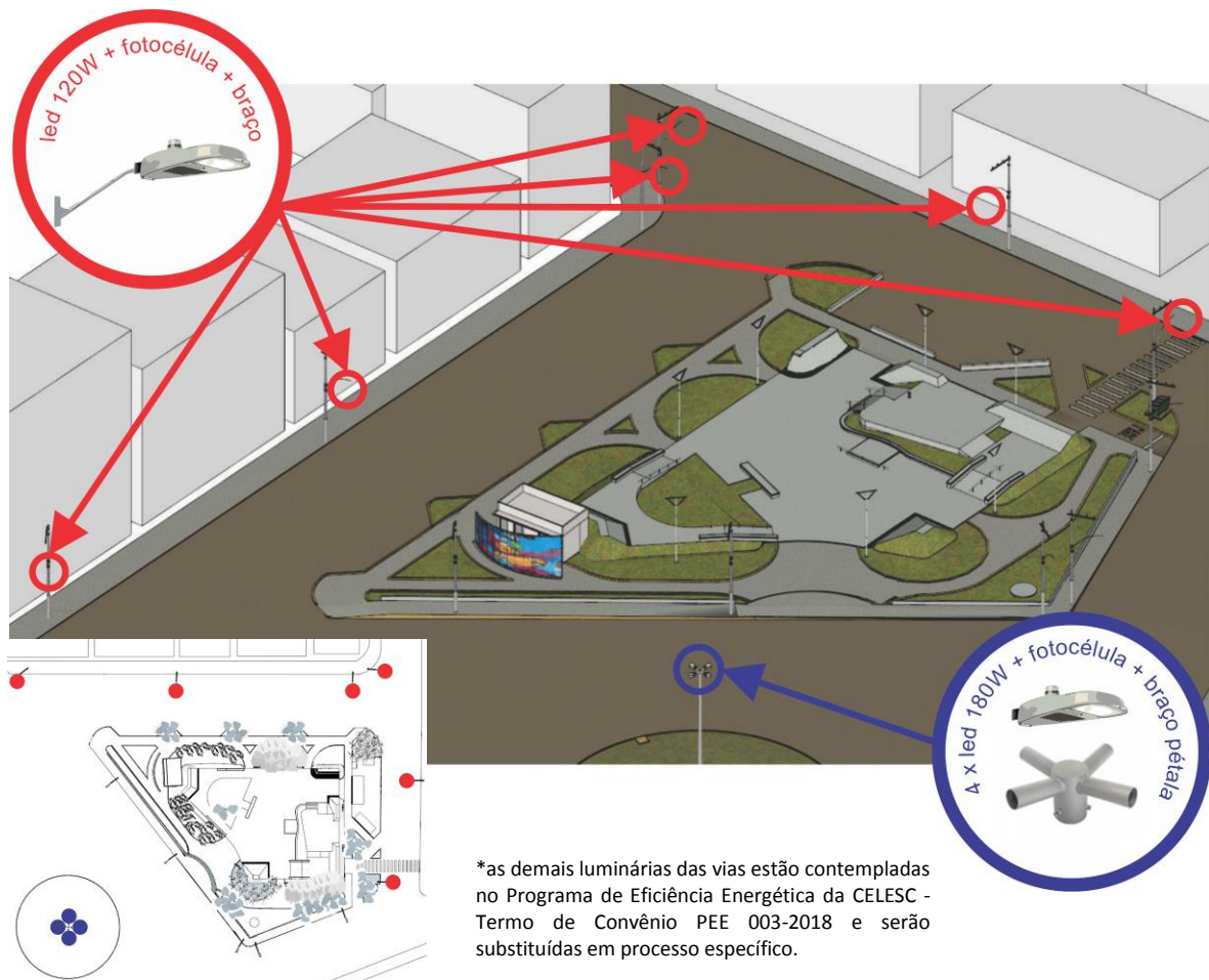
Fig. 6 - Pontos de troca de luminárias nas vias
