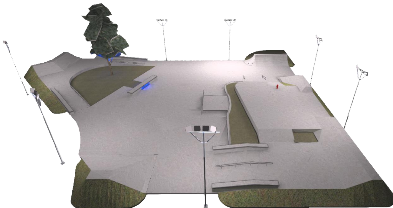
Fig. 3 - Layout do sistema de iluminação da pista de skate
