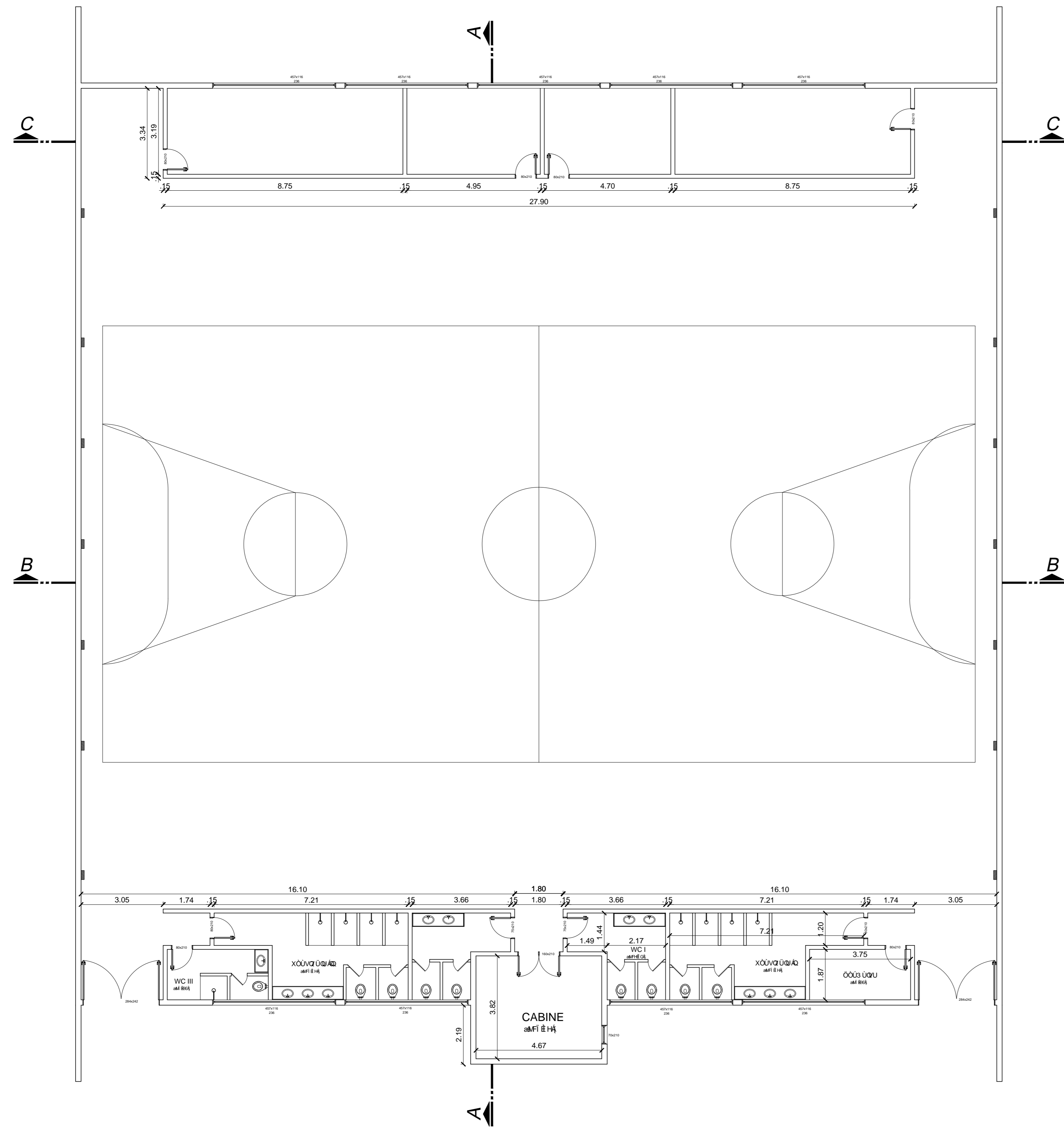
PLANTA BAIXA VESTIÁRIOS/SANITÁRIOS ESC. 1:100 5F95. a
