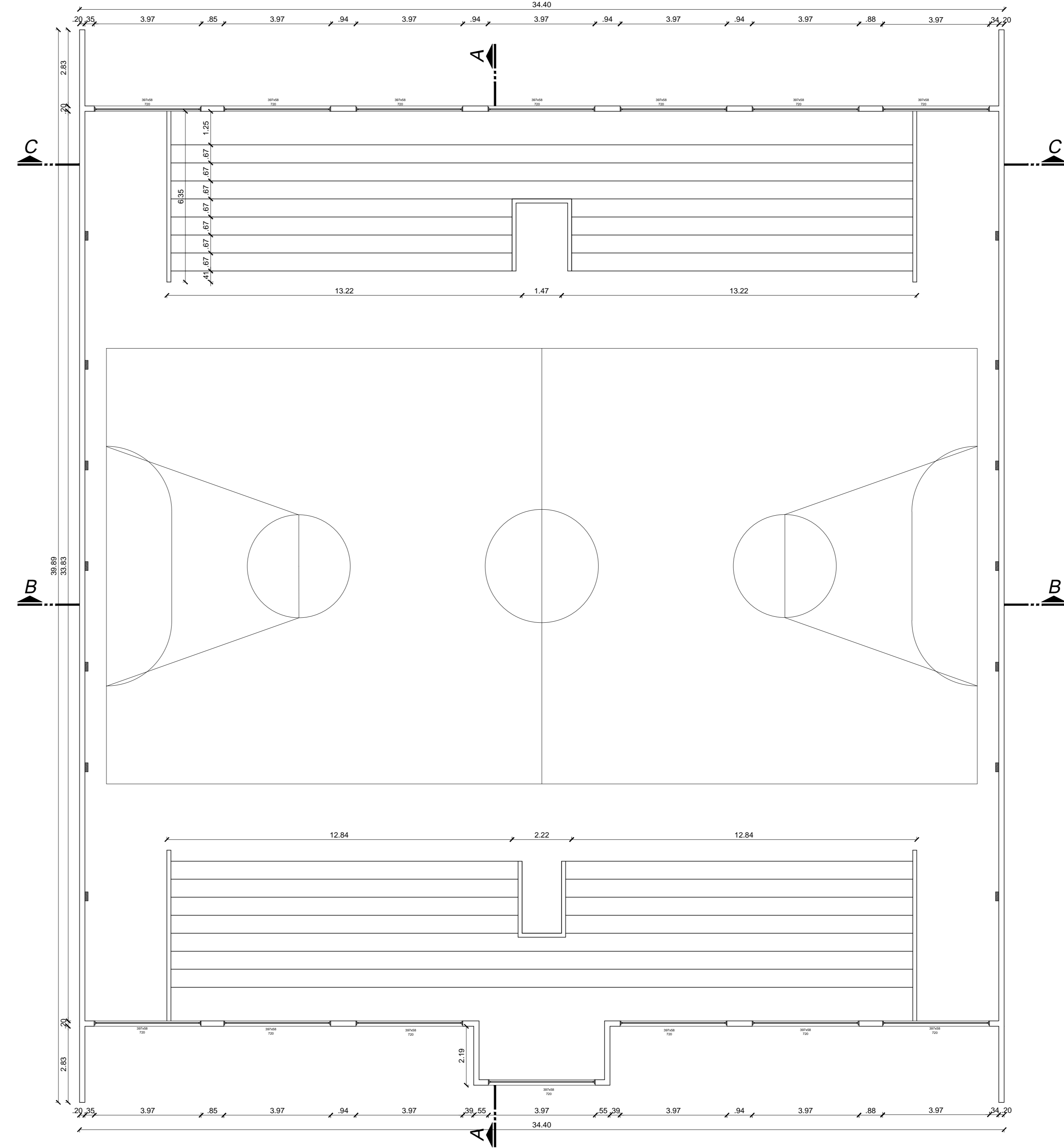
PLANTA BAIXA ARQUIBANCADAS ESC. 1:100 5F95. a
